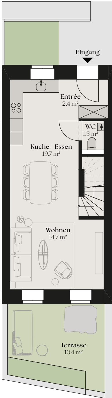
Erdgeschoss
